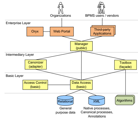
Fig. 1. AProMoRe’s SOA.
